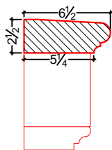
DÉTAIL TYPE 22
