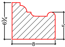
DÉTAIL TYPE 1
