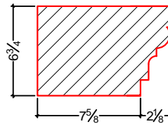
DÉTAIL TYPE CR24
