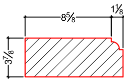
DÉTAIL TYPE CR40
