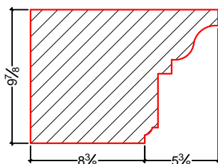
DÉTAIL TYPE CR33
