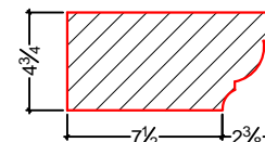
DÉTAIL TYPE CR35
