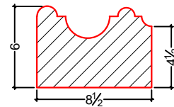
DÉTAIL TYPE 3
