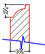
DÉTAIL TYPE 10
