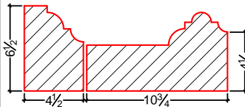
DÉTAIL TYPE 5
