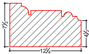
DÉTAIL TYPE 7
