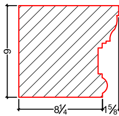
DÉTAIL TYPE CR43
