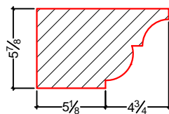
DÉTAIL TYPE CR30
