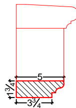
DÉTAIL TYPE 23
