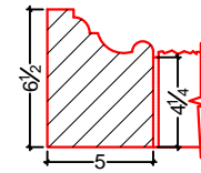
DÉTAIL TYPE 6
