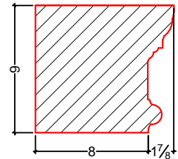
DÉTAIL TYPE CR42
