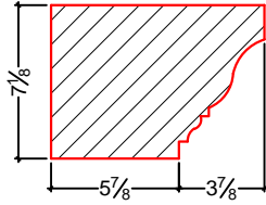
DÉTAIL TYPE CR36
