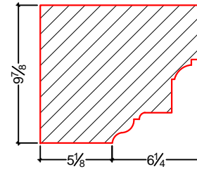
DÉTAIL TYPE CR45
