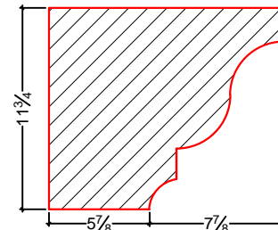
DÉTAIL TYPE CR29
