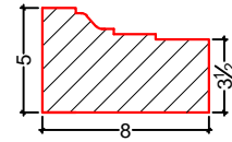
DÉTAIL TYPE 18
