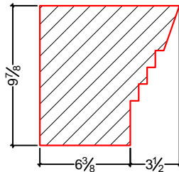
DÉTAIL TYPE CR41
